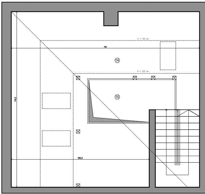
PODDASZE
