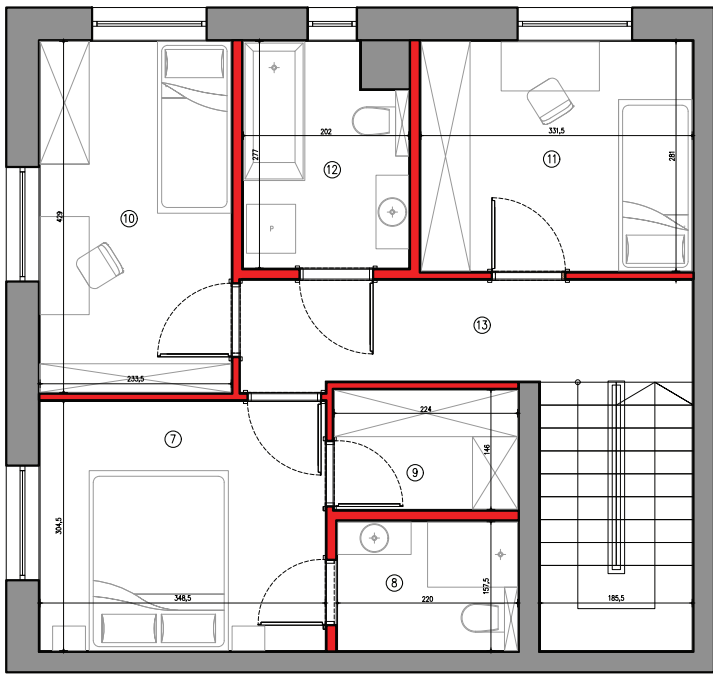
PIĘTRO
